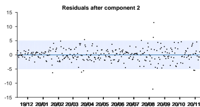
Figure 5: 제 2 경향 요소를 추가한 주가 추정 분포도
