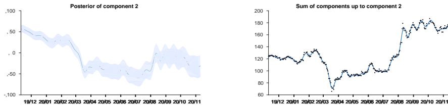
Figure 4: 제 2 경향성의 분포도(왼쪽)과 현재까지 경향성 합 분포와 실제 주가의 비교(오른쪽)
