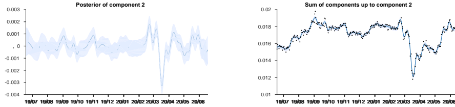
Figure 4: 제 2 경향성의 분포도(왼쪽)과 현재까지 경향성 합인 분포와 실제 선물가격의 비교(오른쪽)
