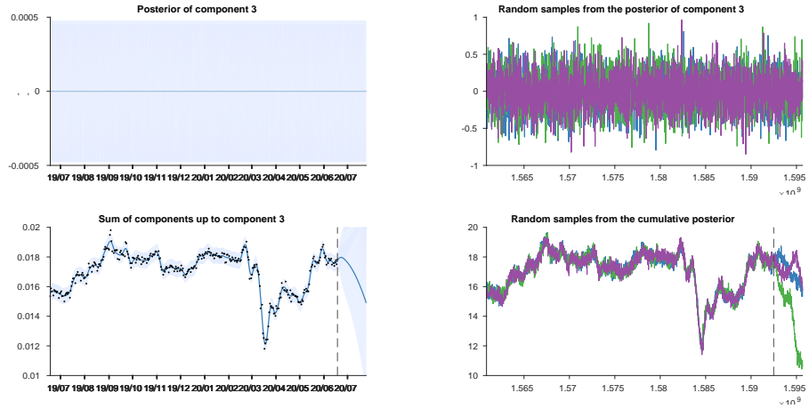
Figure 10: 제 3 경향성의 분포(왼쪽 위)와 현재까지 경향성의 합(왼쪽 아래), 그리고 각 분포에서 추출한 3개의 표본(오른쪽 위, 오른쪽 아래).
