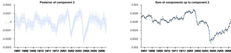
Figure 4: 제 2 경향성의 분포도(왼쪽)과 현재까지 경향성 합이 분포와 실제 선물가격의 비교(오른쪽)
