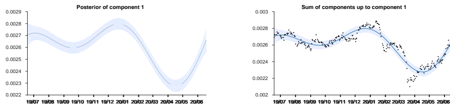
Figure 2: 제 1 경향성의 분포도(왼쪽)과 현재까지 경향성 합인 분포와 실제 선물가격의 비교(오른쪽)
