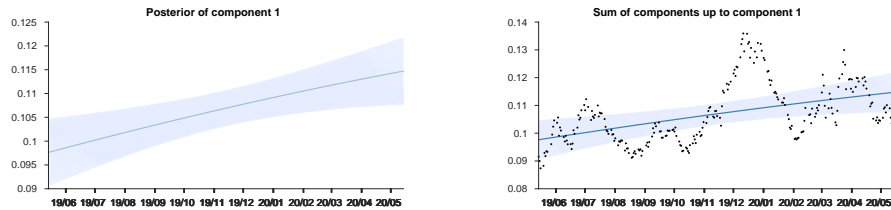
Figure 2: 제 1 경향성의 분포도(왼쪽)과 현재까지 경향성 합인 분포와 실제 요소의 비교(오른쪽)
