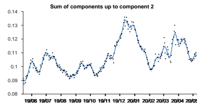
Figure 4: 제 2 경향성의 분포도(왼쪽)과 현재까지 경향성 합 분포와 실제 요소의 비교(오른쪽)
