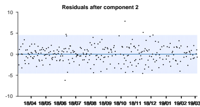
Figure 5: 제 2 경향 요소를 추가한 주가 추정 분포도
